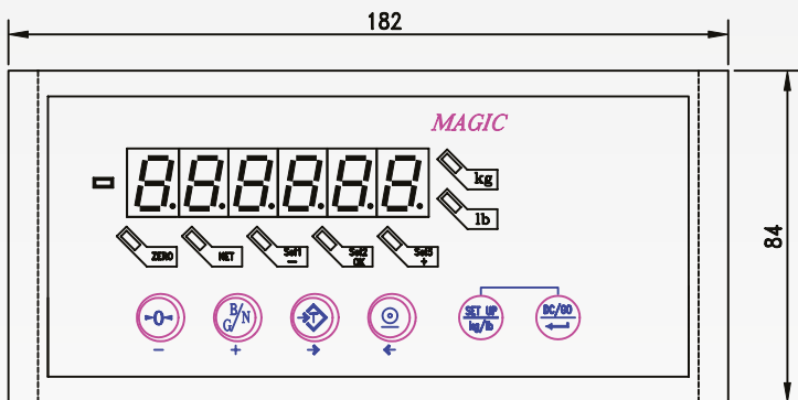
Parte delantera RP15-M Caja ABS
