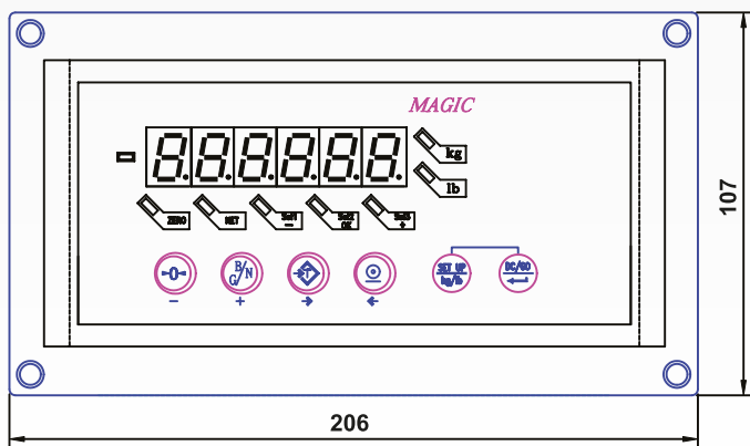
Parte delantera RP15-M Caja INOX
